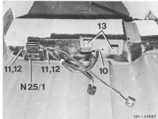
Bild 12 Anordnung Relais Sitzheizung links
