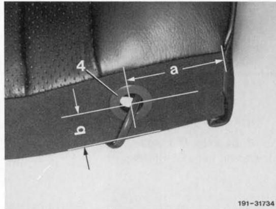
Bild 4 Anordnung Planöse rechter Sitz, links spiegelbildlich a = 80 mm b = 35 mm
