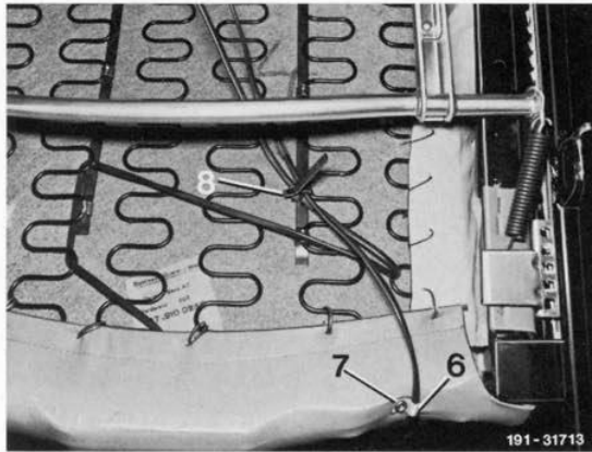
Bild 10 Verlegung elektrische Leitung von Sitzlehne zum Sitzkissen
