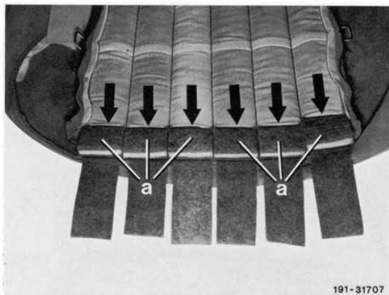
Bild 6 Montage der Heizstreifen an der Lehne oben
