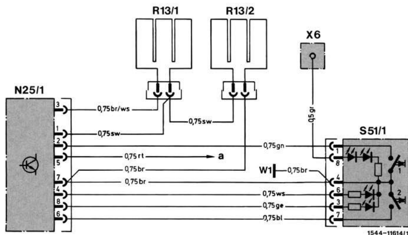
Bild 20 Schaltplan Sitzheizung links, rechts spiegelbildlich
