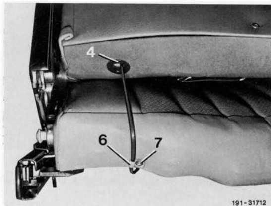
Bild 9 Elektrische Leitungen an Sitzkissenrahmen
