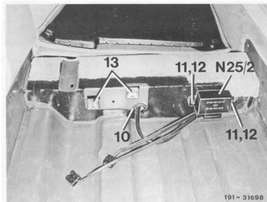
Bild 13 Anordnung Relais Sitzheizung rechts
