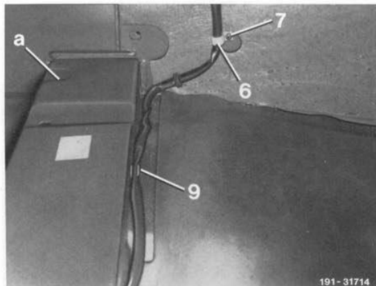
Bild 11 Leitungsverlegung am Querträger rechts, links spiegelbildlich
