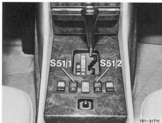
Bild 19 Anordnung Schalter
