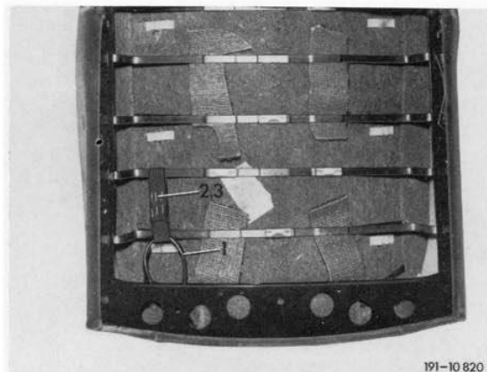
Bild 8 Elektrische Leitungen an Lehnenrahmen
