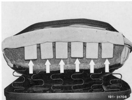
Bild 3 Befestigung Heizkissen an Sitzkissen
