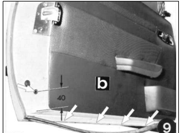
Bohrung in Fahrtür, Halteschiene für Türabdichtungen
