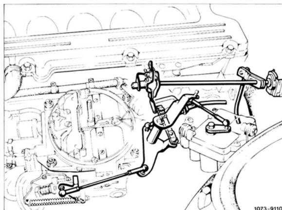
Motor 110 mit Vergaser
