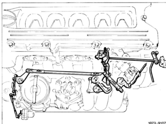
Motor 110 mit KA-Einspritzanlage
